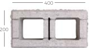
Pustak słupkowy - rozszczepiany z czterech stron
