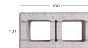
Pustak cały
