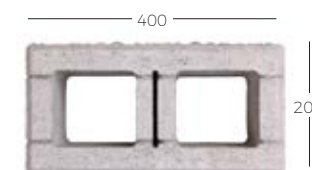
Pustak podmurówkowy
