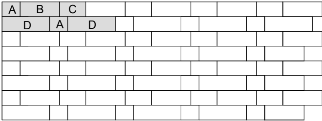
A - 22x18, B - 48x18, C - 32x18, D - 58x18
