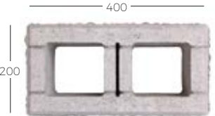
Pustak słupkowy - rozszczepiany z czterech stron
