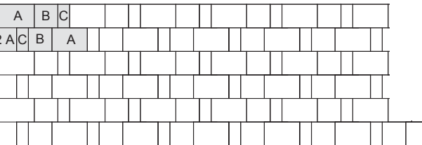
A - 30x20, B - 20x20, C - 10x20
