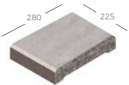
Daszek płaski - rozszczepiany na długości
