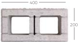
Pustak podmurówkowy - rozszczepiany z dwóch stron
