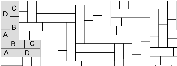
A - 22x18, B - 48x18, C - 32x18, D - 58x18
