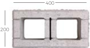
Pustak cały - rozszczepiany z trzech stron
