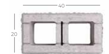
Pustak słupkowy
