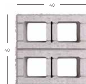
Pustak podwójny
