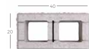
Pustak słupkowy
